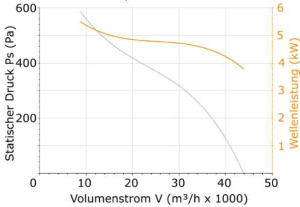
DHPX/SEC-90-4T-7,5
