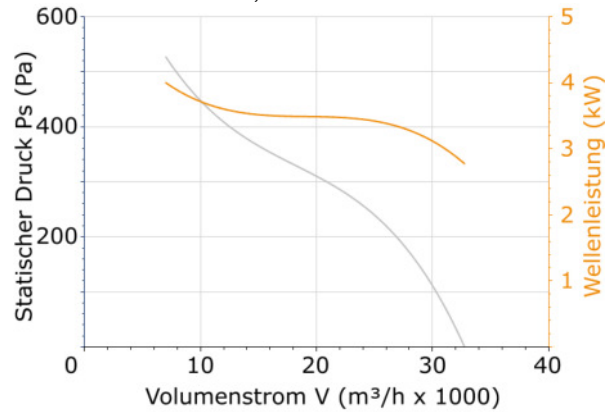
DHPX/SEC-80-4T-5,5
