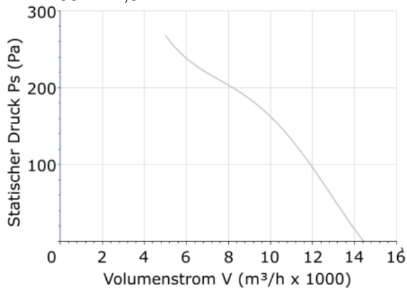
DHPX-56-4T-1,5
