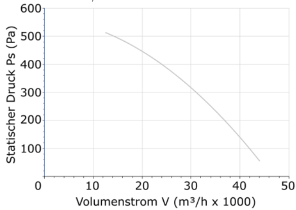
DHPX-90-4T-5,5
