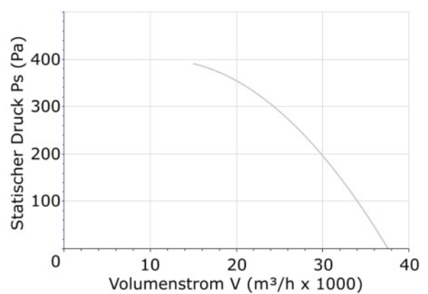
DHPX-80-4T-5,5
