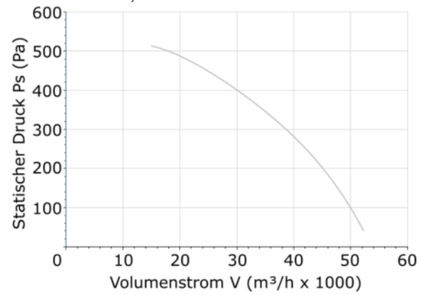
DHPX-90-4T-7,5
