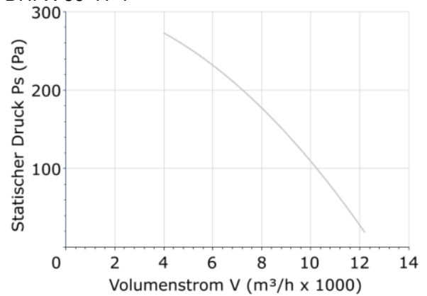
DHPX-56-4T-1
