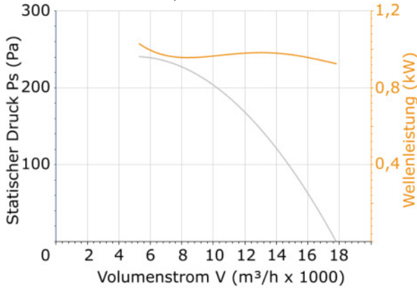
DHPX/SEC-63-4T-1,5
