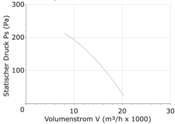
DHPX-71-4T-1,5
