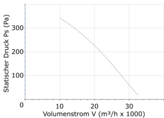
DHPX-80-4T-4
