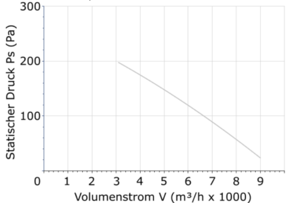
DHPX-50-4T-0,75
