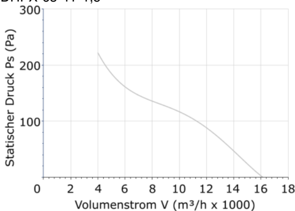
DHPX-63-4T-1,5
