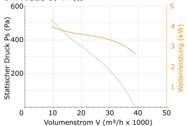
DHPX/SEC-90-4T-5,5
