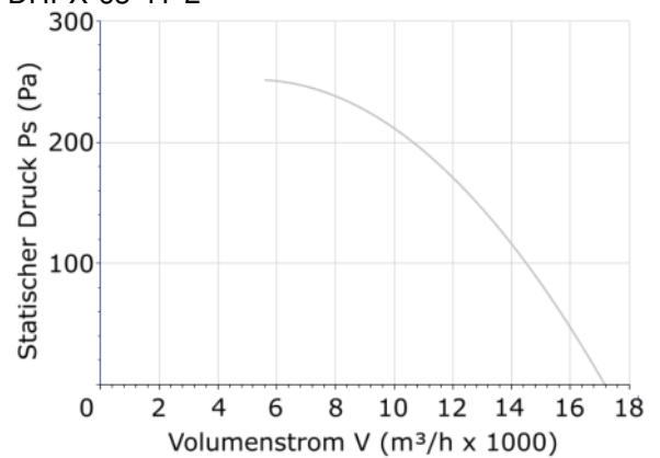
DHPX-63-4T-2
