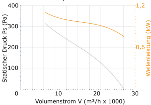
DHPX/SEC-71-4T-1,5
