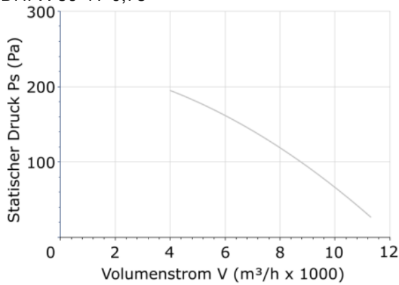
DHPX-56-4T-0,75
